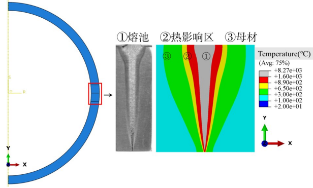
图 6 焊接接头组织成分分布区域
