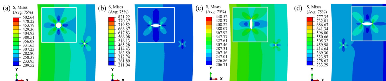
图 8 不同形状及位置的内部缺陷 Von Mises 应力分布
