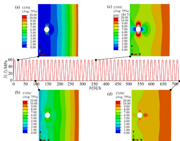
图 12 循环载荷下, 圆形气孔氢浓度的演变过程
