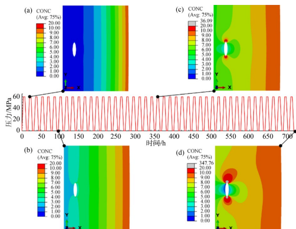
图 13 循环载荷下, 椭圆形气孔(横向)氢浓度的演变过程
