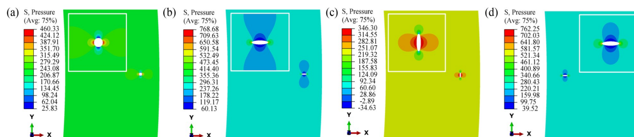
图 9 不同形状及位置的内部缺陷等效压应力分布
