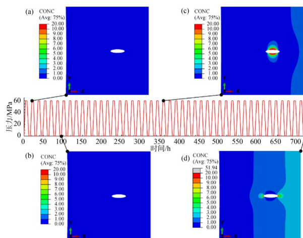
图 14 循环载荷下, 椭圆形气孔(垂向)氢浓度的演变过程
