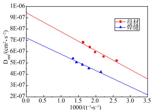
图3 Ti6Al4V 合金的母材和焊缝的 D_{app}-1000/t 曲线
