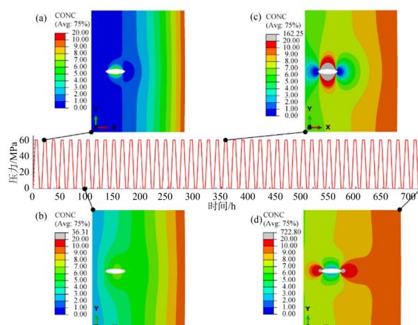
图 15 循环载荷下, 椭圆形气孔(横向)氢浓度的演变过程
