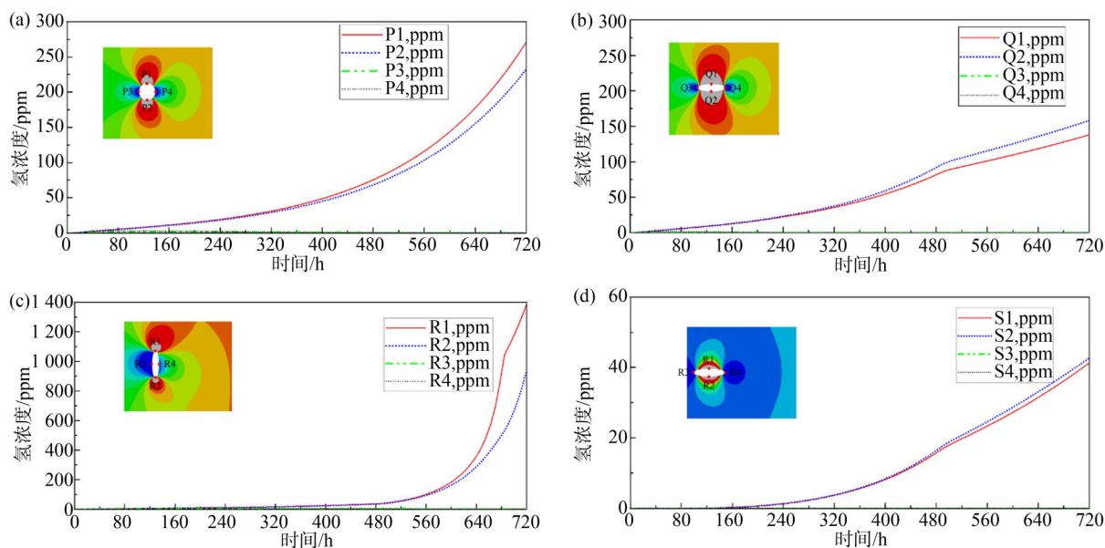
图 11 内部缺陷处,静态加载下氢浓度的变化
