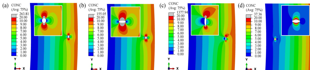
图 10 不同形状及位置的内部缺陷处氢浓度分布
