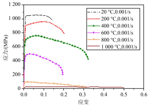
图 5 Ti6Al4V 随温度变化的应力-应变曲线 [11]
