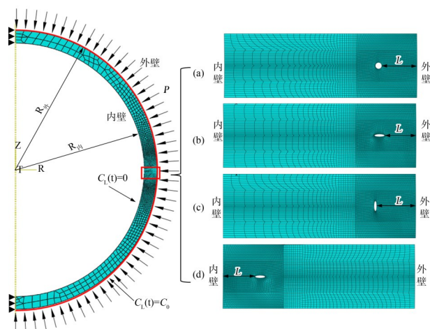
图7 耐压球壳及焊缝处的内部缺陷示意
