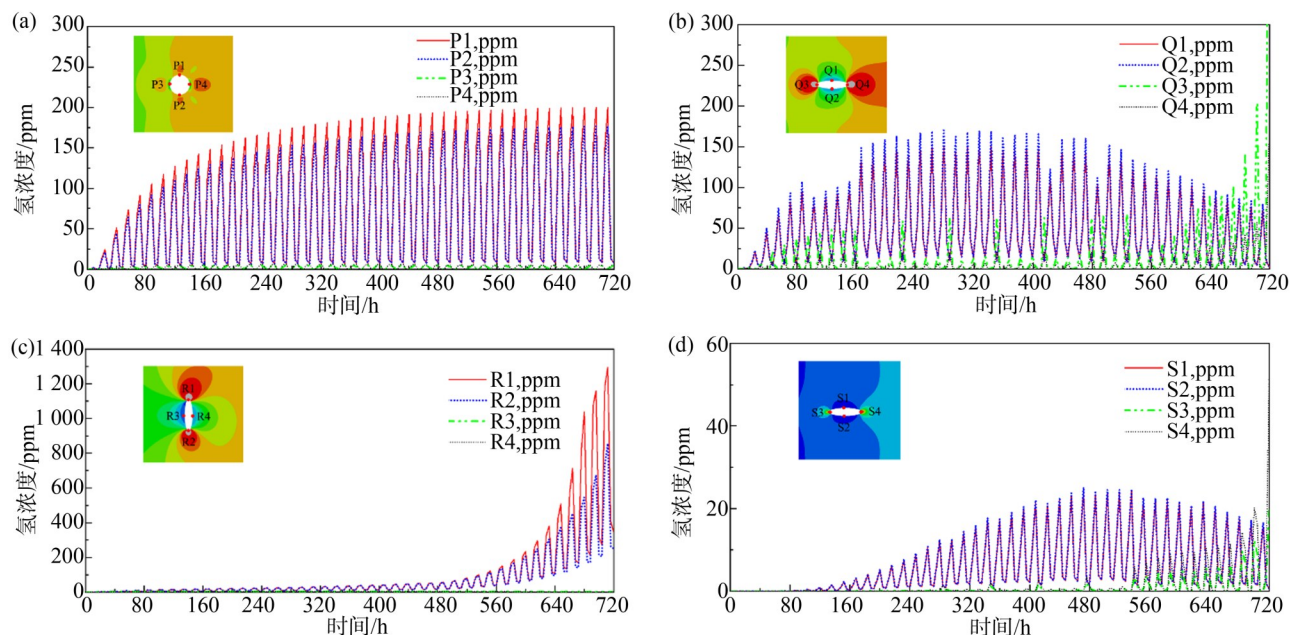
图 16 内部缺陷处,动态加载下氢浓度随时间的变化
