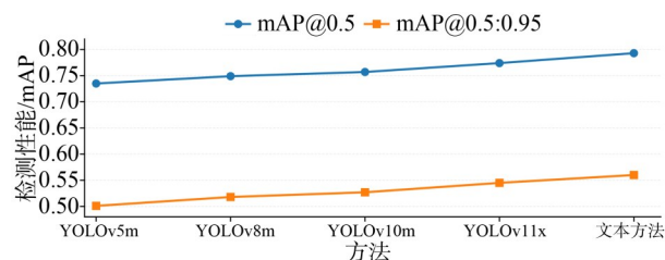
图6 各模型检测性能对比
