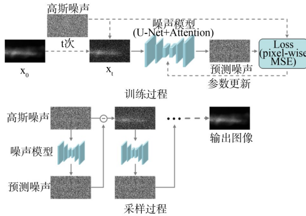
图2 DDPM模型训练和采样过程
