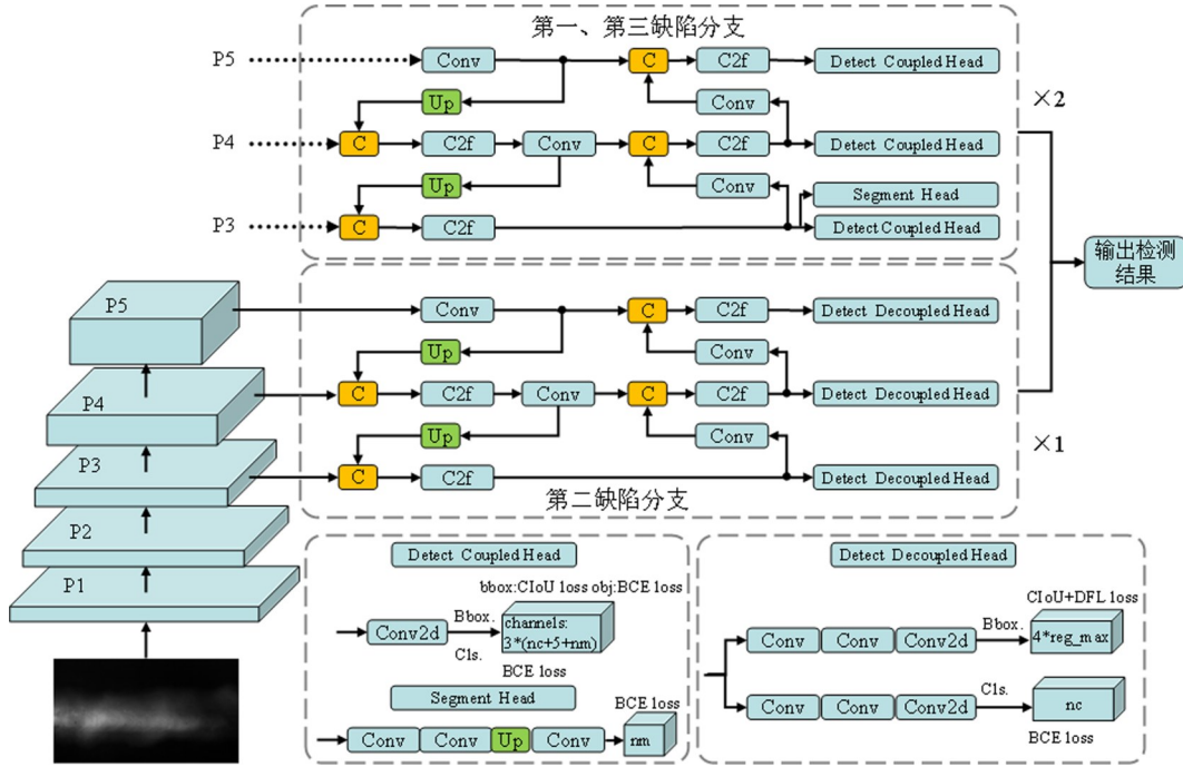
图 3 核电厂领域焊缝缺陷检测模型结构
