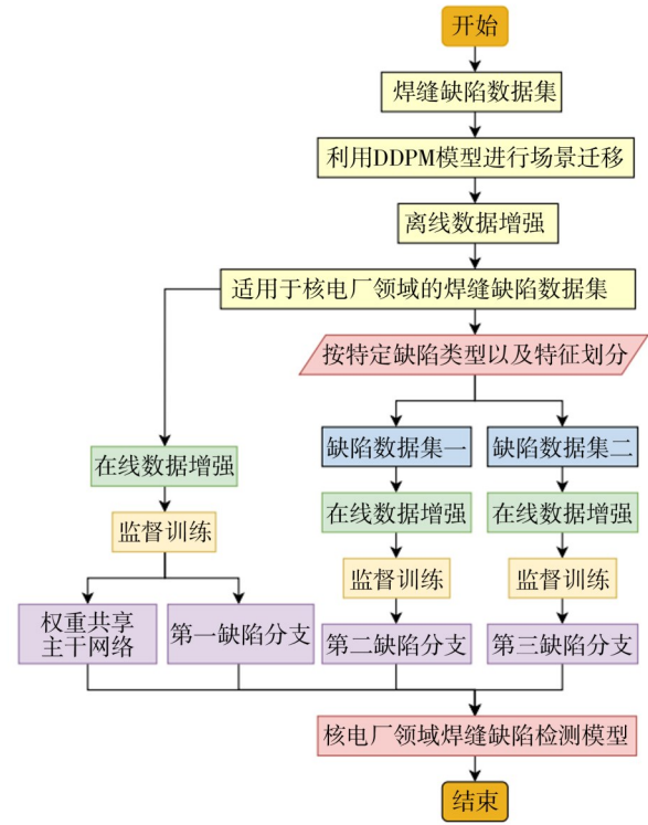
图 1 核电厂焊缝缺陷检测模型训练流程
