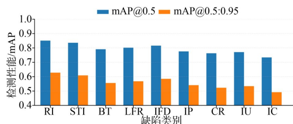
图5 各类别缺陷检测性能并列柱状图
