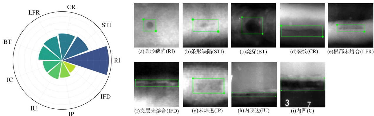
图4 长输管线场景下9类焊缝缺陷实例数量分布及示例
